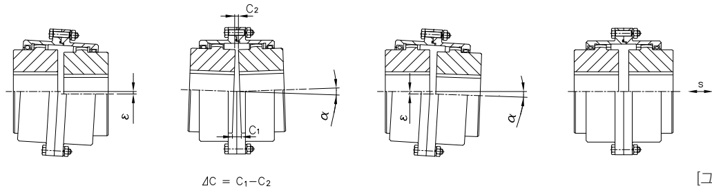
평행오정렬량( \epsilon, \epsilon' )과 허브의 면간거리 편차량( \Delta C ), 축방향 변위량( S ) - (NGG타입)
